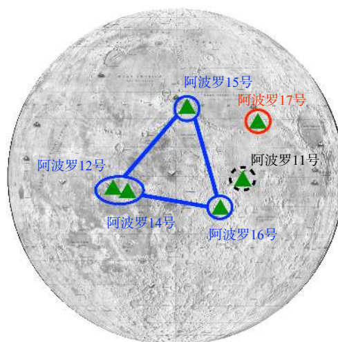
图 1 阿波罗月面着陆点的位置分布图(修改自 Nunn et al., 2020).被动月震实验(PSE)是在阿波罗 11、12、14、15 和 16 号站进行的(11 号站只运行了大约 3 个星期).第一种主动月震实验(ASE)设在 14 和 16 号站.第二种主动实验,也称为月球表面剖面实验(LSPE),设在 17 号站.17 号站还包括月球表面重力仪(LSG),能够提供额外的被动月震信息
