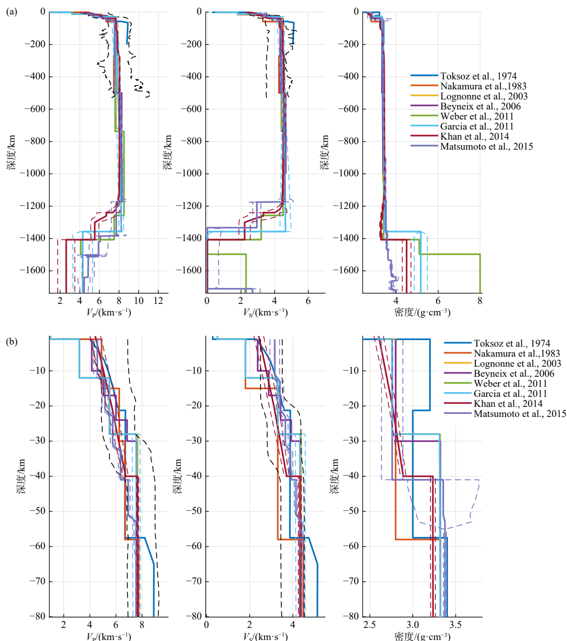
图 4 2019 年以前发表的月球速度和密度模型的比较 (修改自 Garcia et al., 2019). (a) 从月球表面到月球中心的 P 波速度、S 波速度和密度的径向剖面; (b) 月球和月幔上部的局部放大图. 实线表示每个研究的平均值或最可能的模型, 虚线表示可用的一个标准偏差误差栏. 黑色虚线表示等值线, 包括 Khan 和 Mosegaard (2002) 中概率密度最高的模型分布的一半, 仅限于月球的前 500 km
